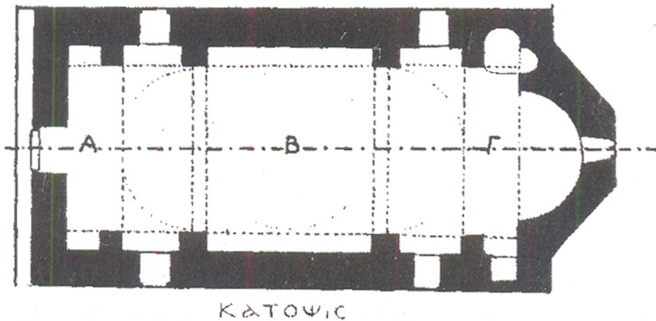
Κάτοψη του καθολικού. Σχέδιο Ματίνας Καβουρίνου.
