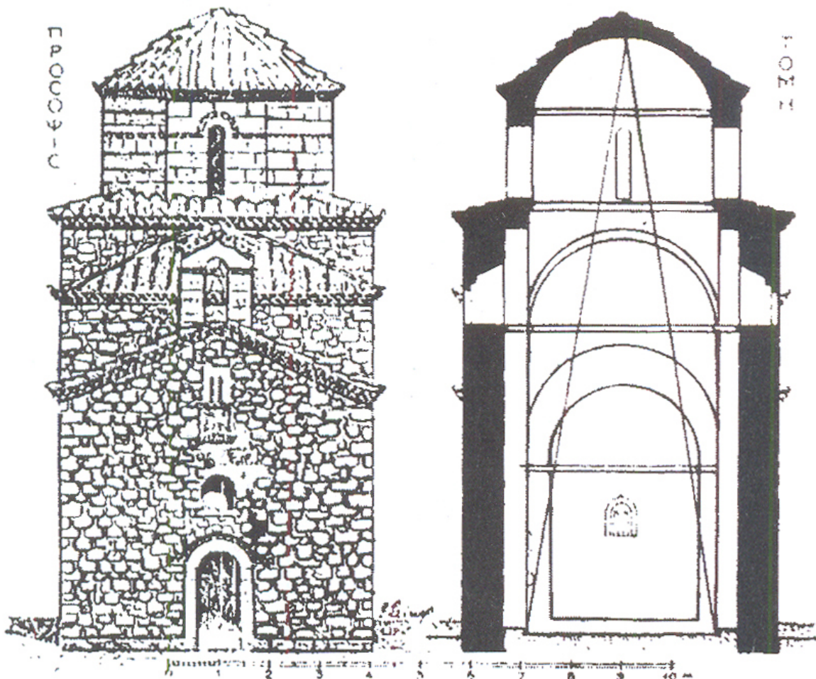
Πρόσοψη και κατά πλάτος τομή του καθολικού. Σχέδια Ε. Στίκα.
