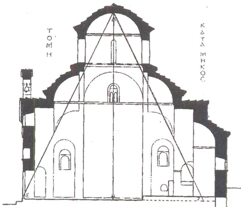
Κατά μήκος τομή του καθολικού. Σχέδιο Ε. Στίκα.
