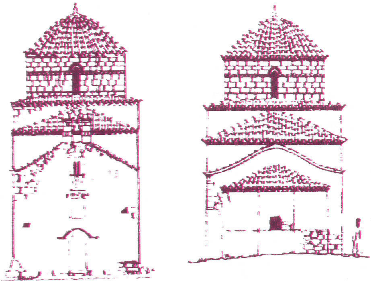
Δυτική και Ανατολική όψη καθολικού. Σχέδια Γ. Δούσκα.
